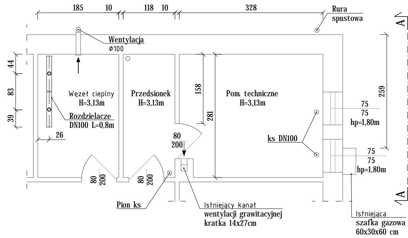
RZUT WĘZŁA CIEPLNEGO I POM TECHNICZNEGO SKALA 1:50
