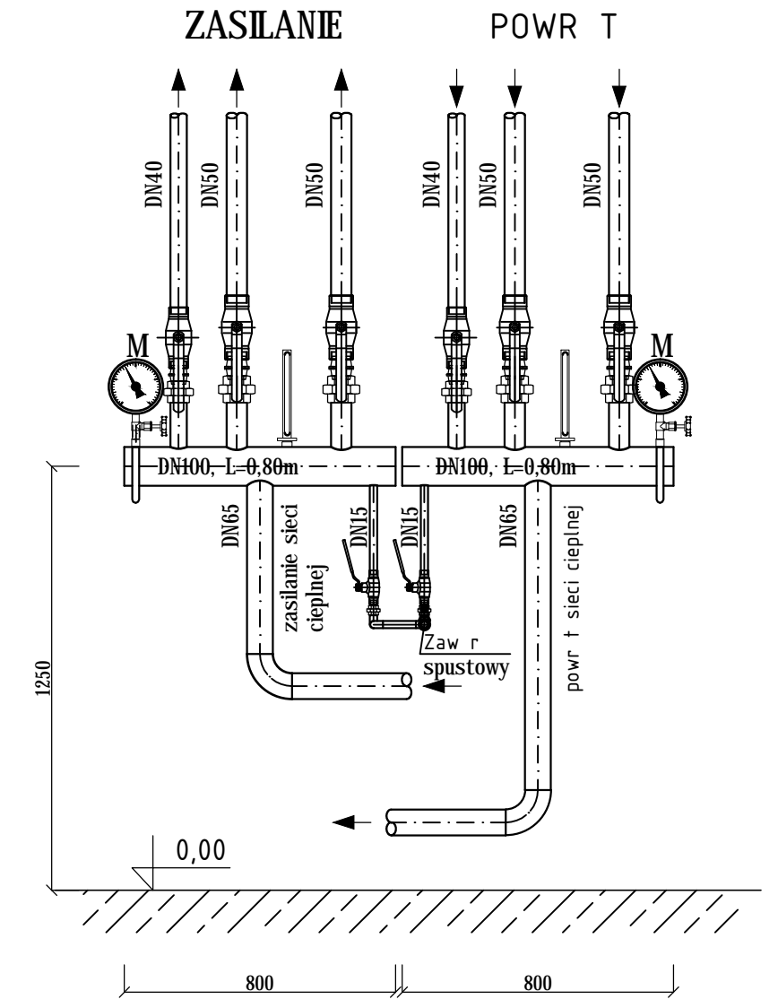
ROZDZIELACZ C.O. SKALA 1:20
