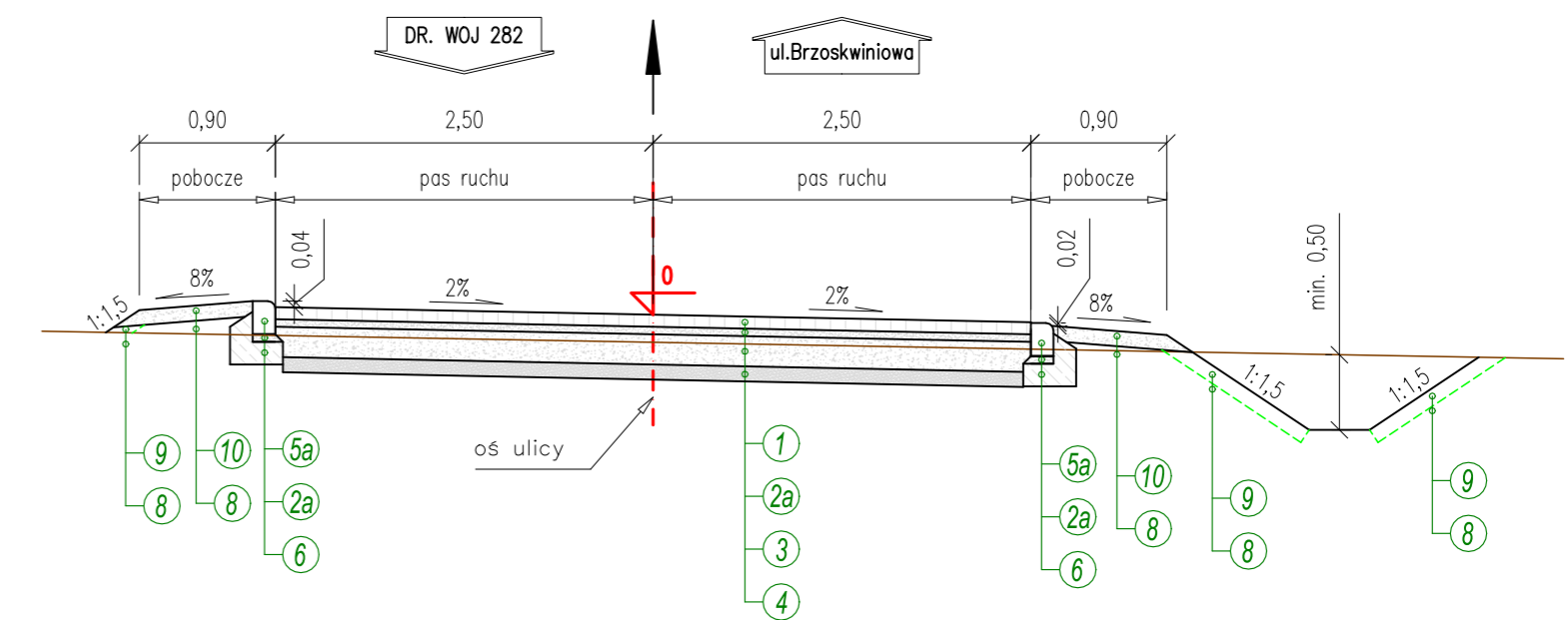
PRZEKRÓJ NORMALNY NR 2 droga gminna NR 007008F - ul. Brzskwiniowa km 0+280,00 ÷ km 0+579,28
