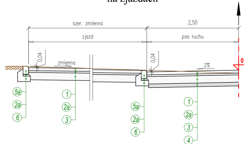
PRZEKRÓJ NORMALNY NR 4 na zjazdach
