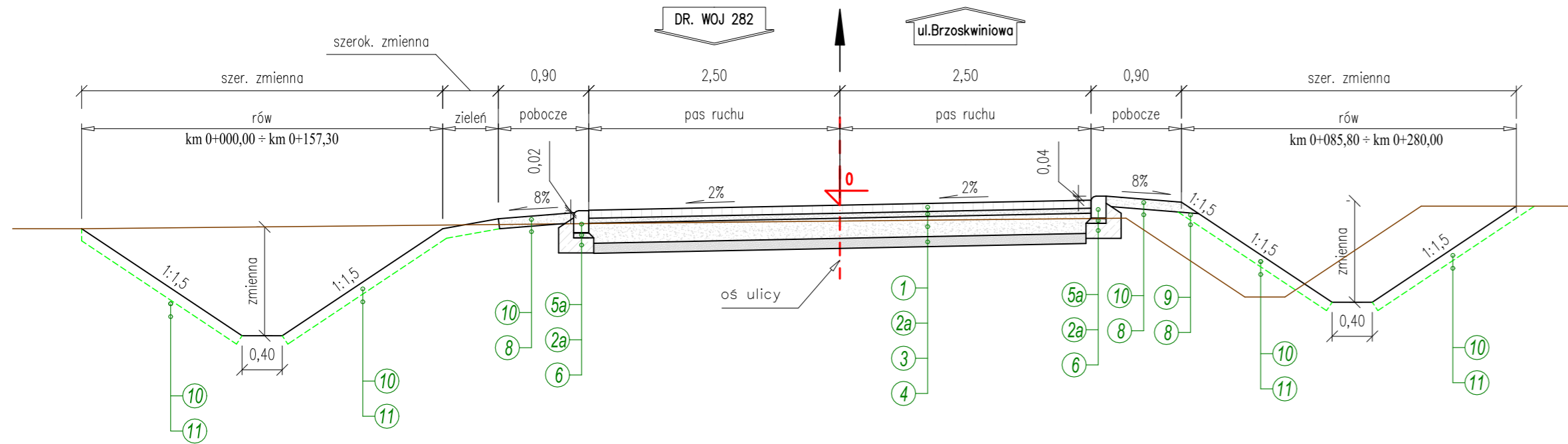
PRZEKRÓJ NORMALNY NR 1 droga gminna NR 007008F - ul. Brzskwiniowa km 0+000,00 ÷ km 0+280,00
