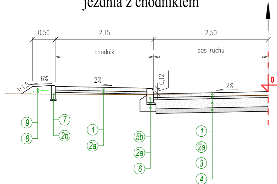
PRZEKRÓJ NORMALNY NR 3 jezdnia z chodnikiem
